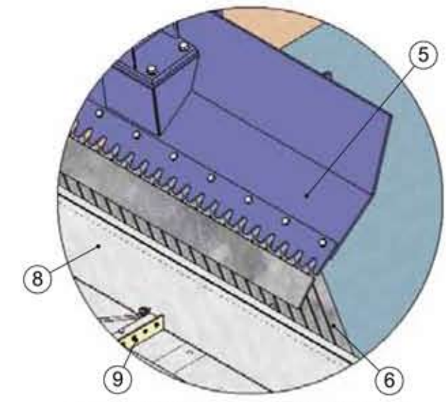
ГРЕБЕНЬ В КОНЦЕ ПОДЪЕМА
