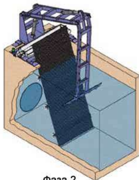
Фаза 2 Движение вниз без прочесывания
