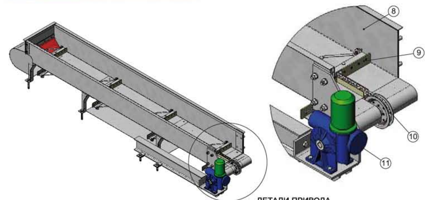
ДЕТАЛИ ПРИВОДА ГРЯЗЕУЛОВИЕТЯ
