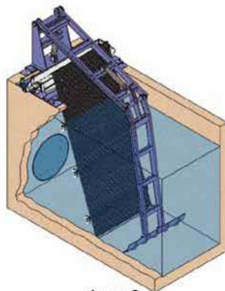
Фаза 3 Крайне нижнее положение
