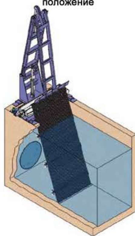
Фаза 6 Крайне верхнее положение
