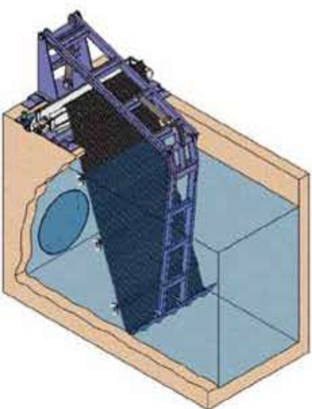
Фаза 4 Начало подъема
